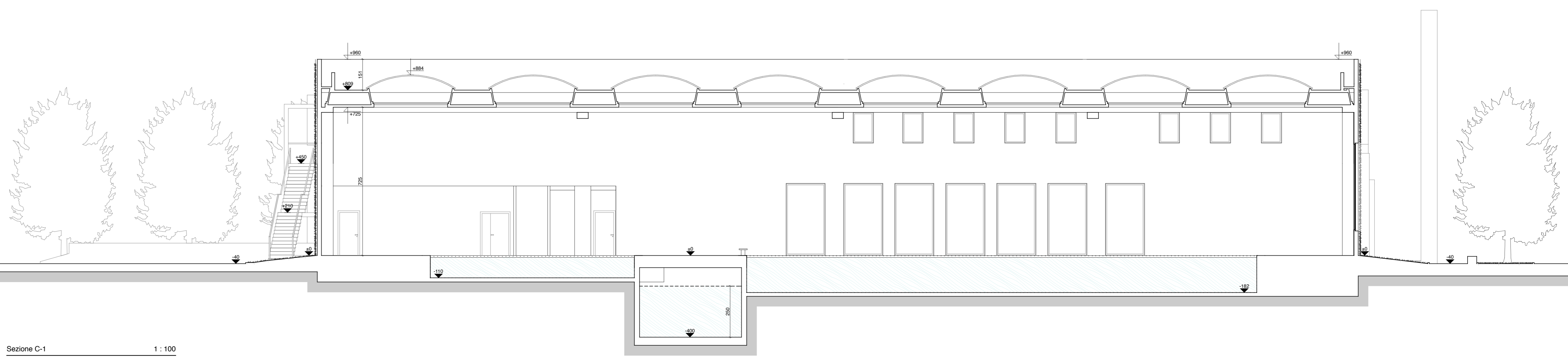
Sezione C-1 1 : 100
