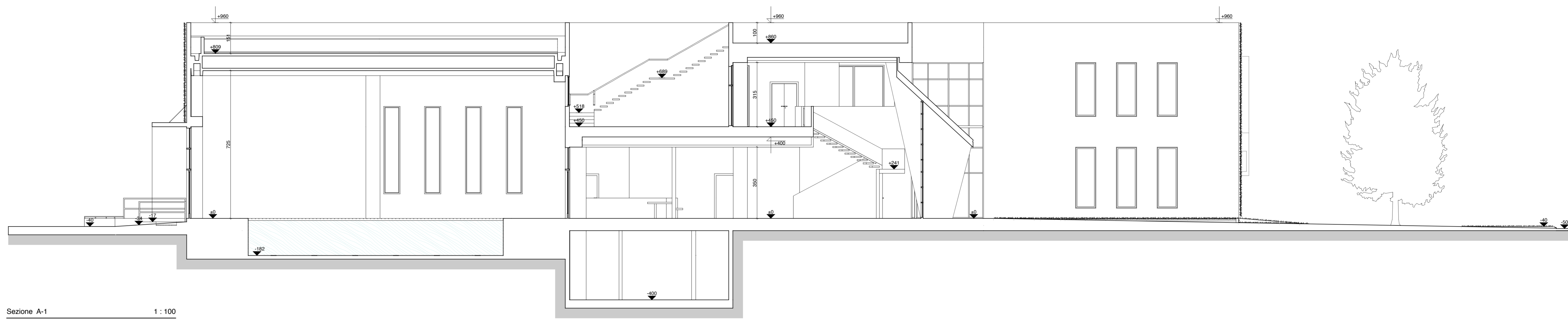
Sezione A-1 1 : 100
