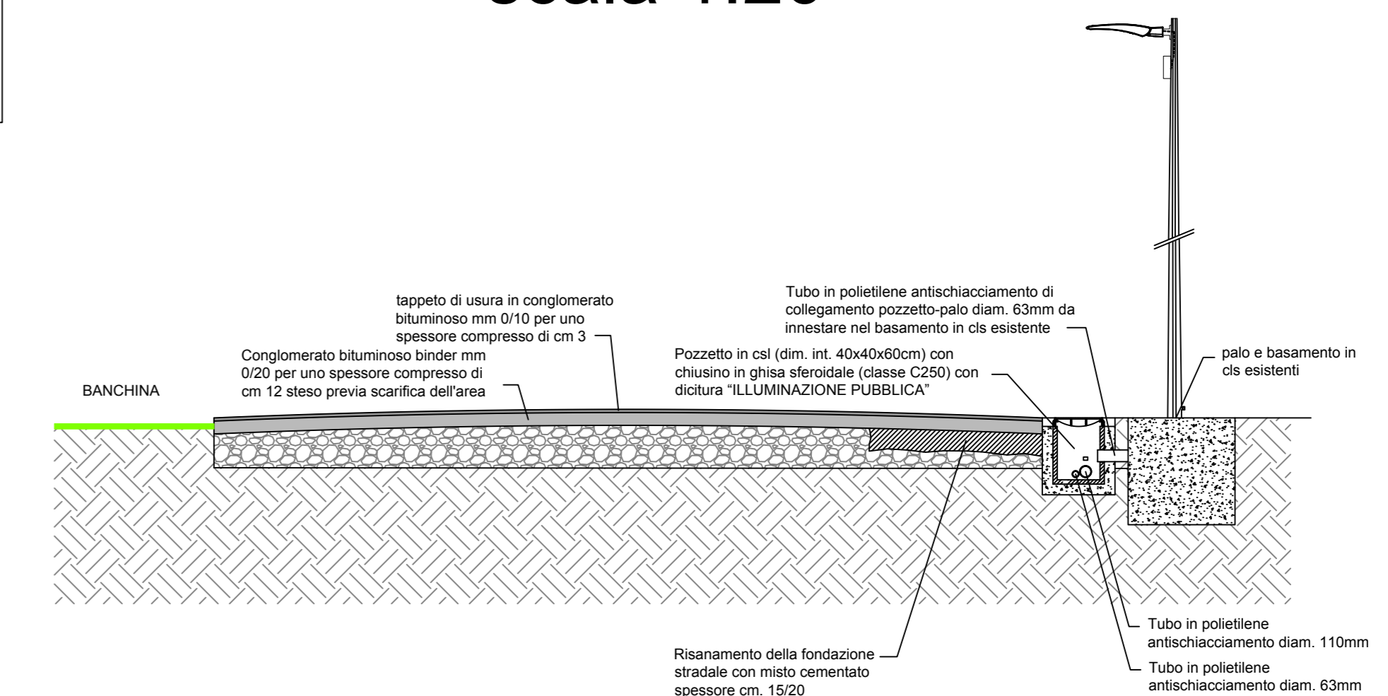
SEZIONE TIPO scala 1:20
